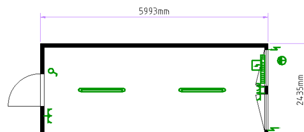
Verbindungscontainer 19'x8'
